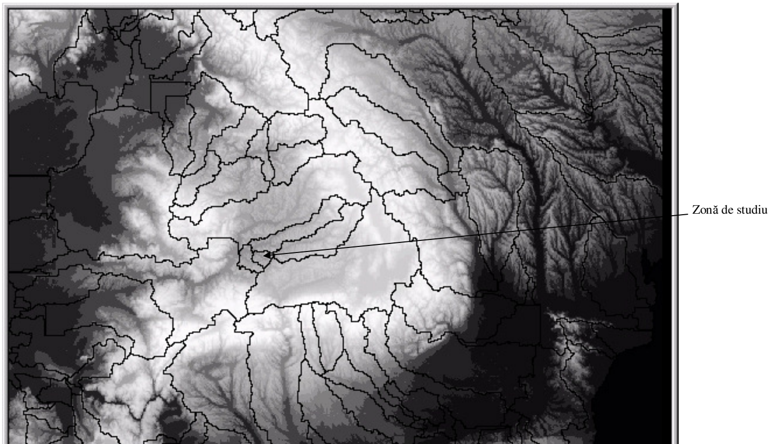
Figura 2 Modelul Numeric de Teren al României rezultat din "GTOPO30" cu suprapunerea bazinelor de drenaj definite pe baza acestuia în "HYDRO 1K". Altitudinile sunt codificate în tonuri de gri, de la nuanțe închise pentru altitudini joase, la nuanțe deschise pentru cele înalte
